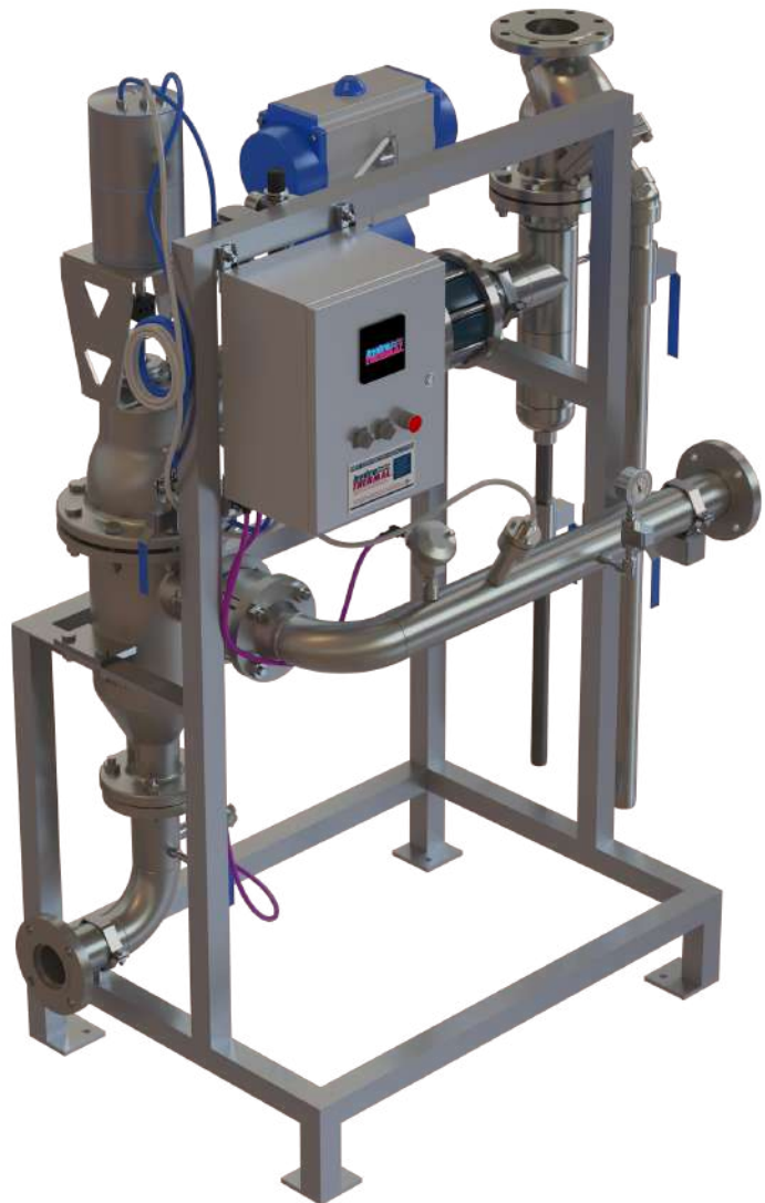
EZ Heater Skid
